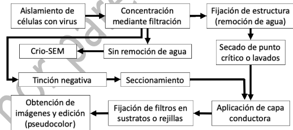
Fig 3. Esquema de preparación de muestras para uso en microscopía electrónica de barrido y transmisión. Fuente: elaboración propia.
