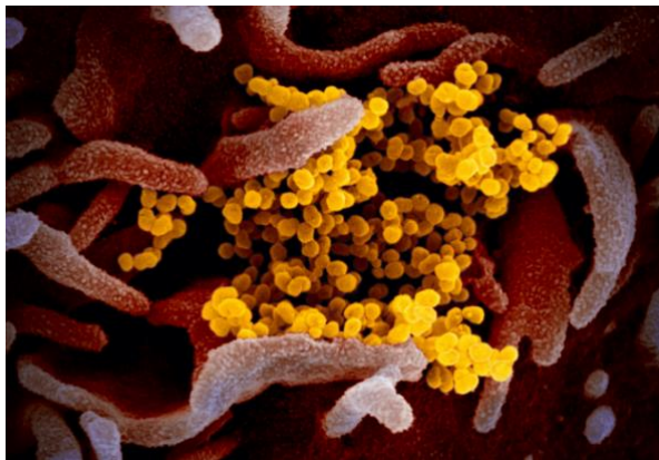
Fig 1. Micrografía electrónica de barrido (SEM) de SARS-CoV-2 (en Amarillo) extraído de un paciente contagiado en EEUU, emergiendo de la superficie de las células (en lila) cultivadas en el laboratorio. Imagen del Rocky Mountain Laboratories (RML) del National Institute of Allergy and Infectious Diseases (NIAID).
